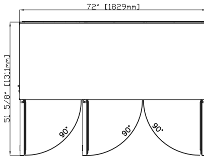
EDWR(F)72-B Top
