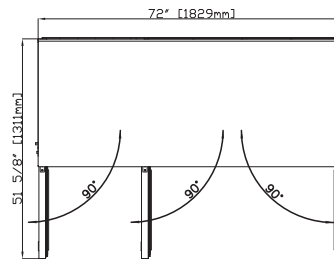
EDWR(F)72-B Top
