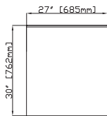
EDWR(F)27-B Top
