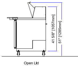
Open Lid
