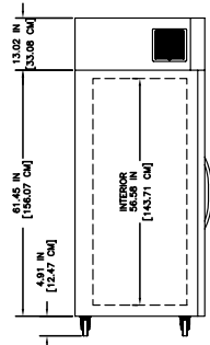
TYP. LEFT END VIEW
