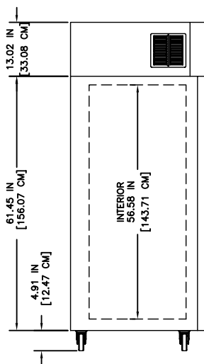
TYP. LEFT END VIEW
