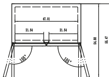
C-49RM-HC TOP VIEW
