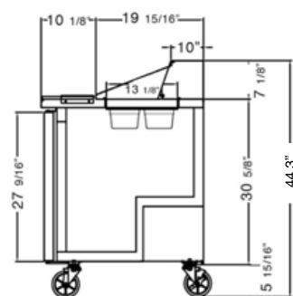
SIDE VIEW(1,2,3)
