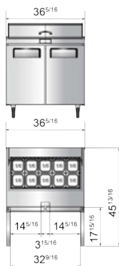
MSF3610GR
