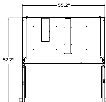
EDJR-49-B TOP EDRF-49-B TOP
