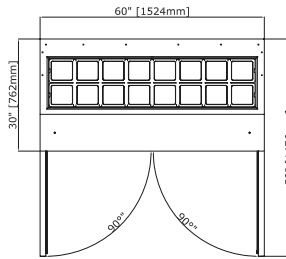
EDST60-16-B Top
