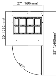
EDST27-8-B Top
