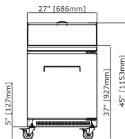
EDST27-8-B Front
