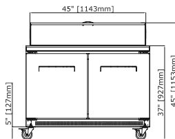
EDST48-12-B Front
