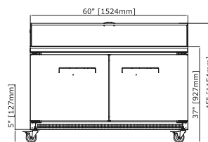
EDST60-16-B Front
