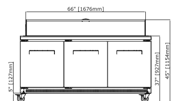
EDST72-18-B Front
