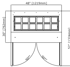
EDST48-12-B Top
