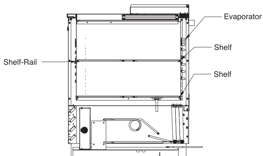
TBC-24S*-GF-N#
